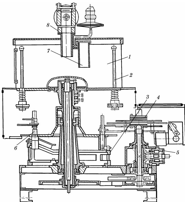
Рис. 1.101. Автомат-наповнювач ДН1
