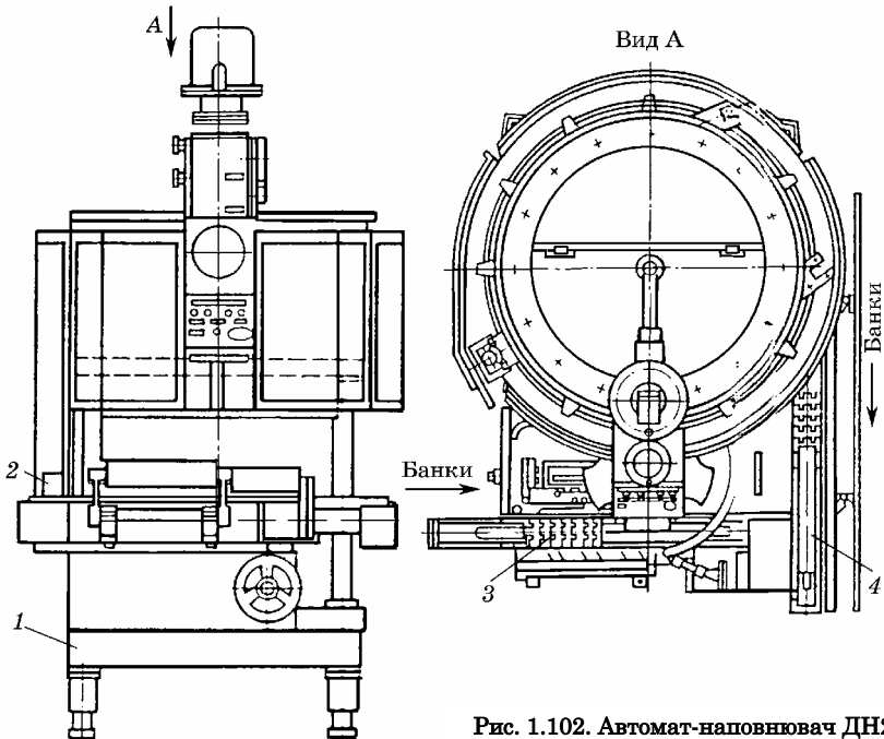
Рис. 1.102. Автомат-наповнювач ДН2
