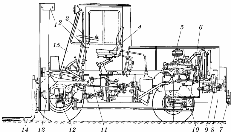
Рис. 4.17. Автовантажувач 4014
