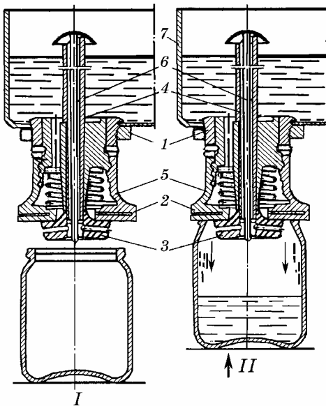
Рис. 1.100. Пристрої для дозування за рівнем
