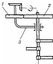
Рис. 1.53. Планетарна мішалка:
