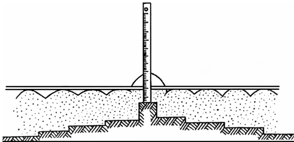
Рис. 71. Вимірювання висоти складного гребеня і глибини оранки під ним
