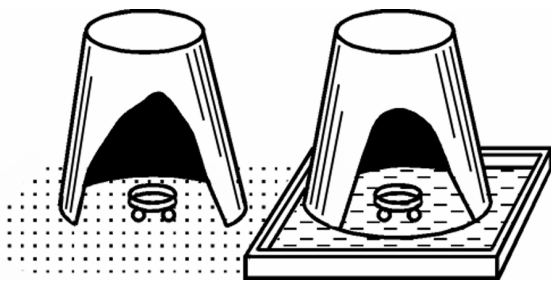
Рис. 10. Прилад для визначення кількості вуглекислого газу, що виділяється з ґрунту (метод В.І. Штатнова)
