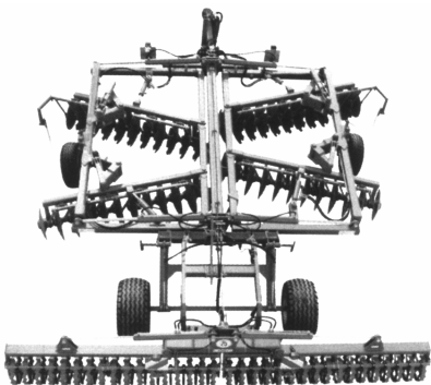
Рис. 65. Дискова борона EURODISC
