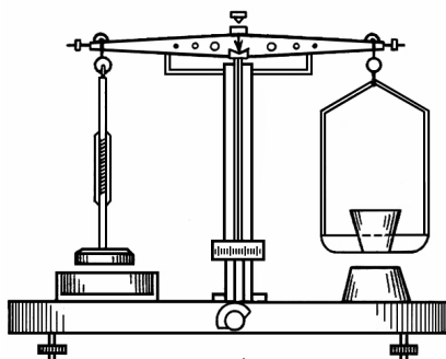
Рис. 2. Прилад М.А. Качинського для визначення липкості ґрунту
