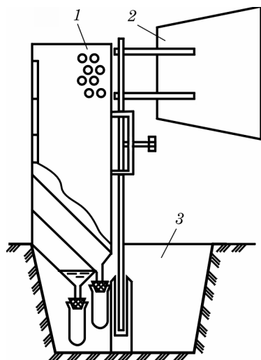
Рис. 13. Пиловловлювач УПЗ-50
