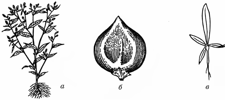
Рис. 19. Гірчак шорсткий: а — рослина; б — насінина; в — сходи
